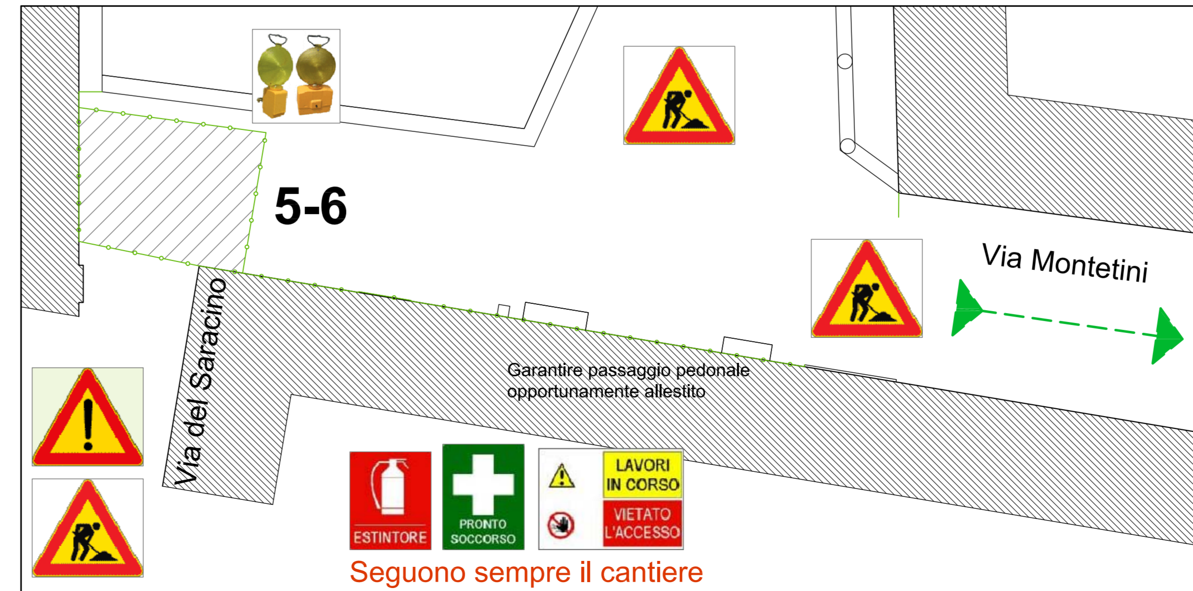
Sottofase 1 - FASE 3 Chiusura temporanea accesso da via del Saracino max 1 gg
